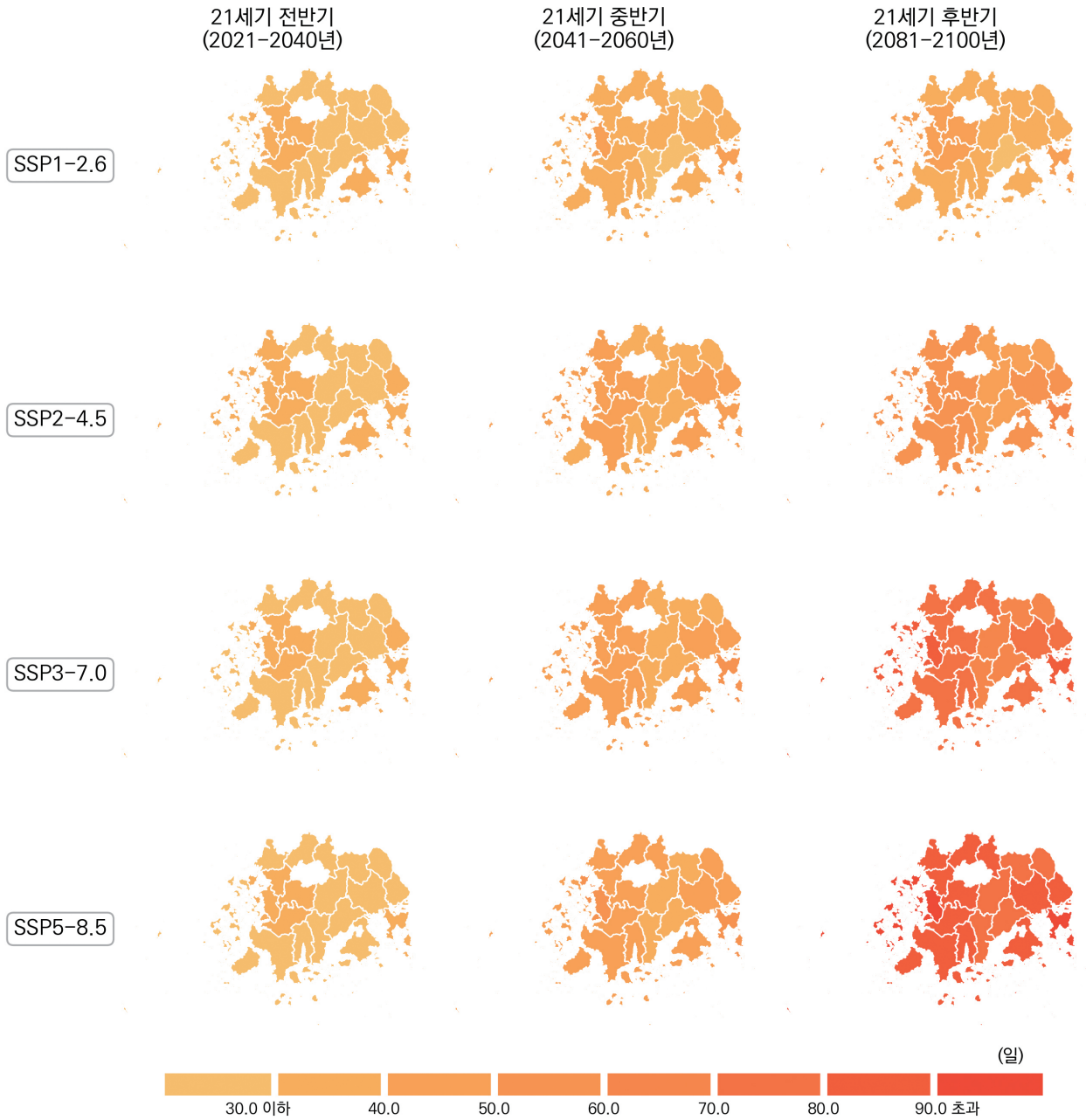
그림 4-19. 전라남도의 열대야일수(일) 전망 분포도
