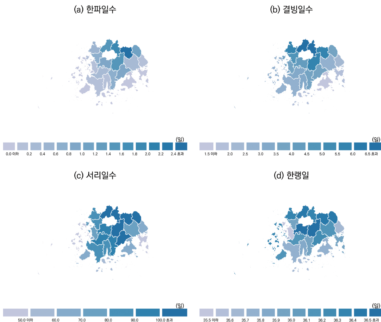
그림 3-3. 현재(2000-2019년) 전라남도 저온 관련 극한기후지수 분포
