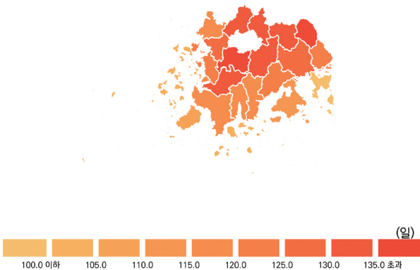
그림 3-2. 현재(2000-2019년) 전라남도 고온 관련 극한기후지수 분포
